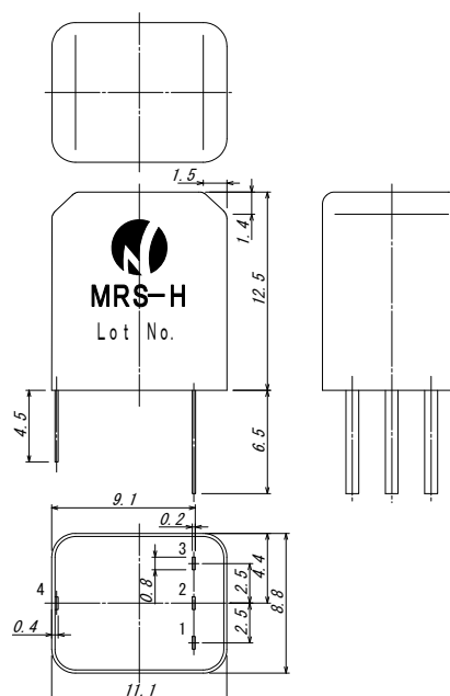
外形図
